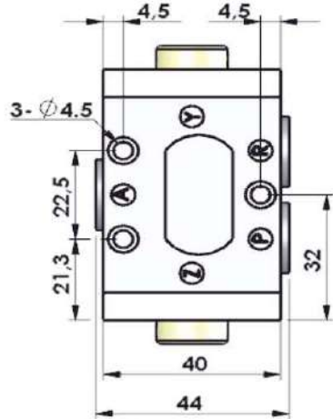
TPY-32 Normalde açık Normally open
