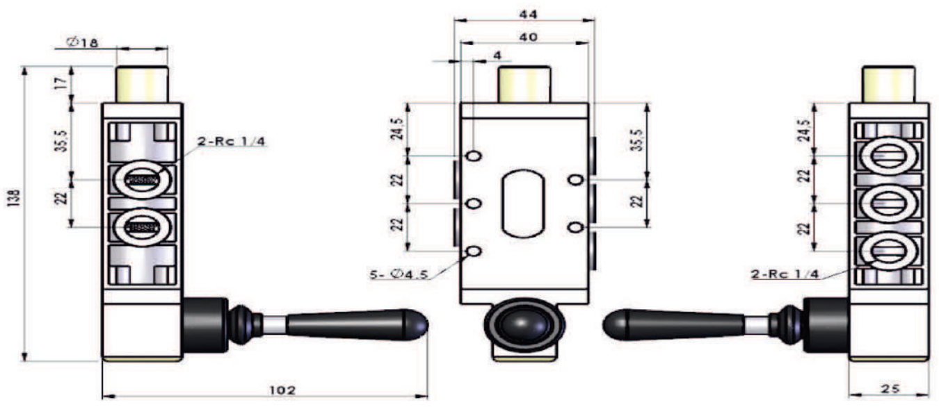
TKYK-53/A Normalde Açık Normally Open
