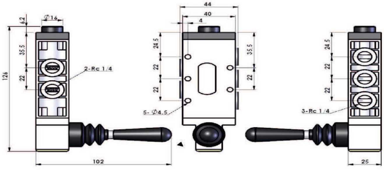
TKSK-53/A Normalde Açık Normally Open
